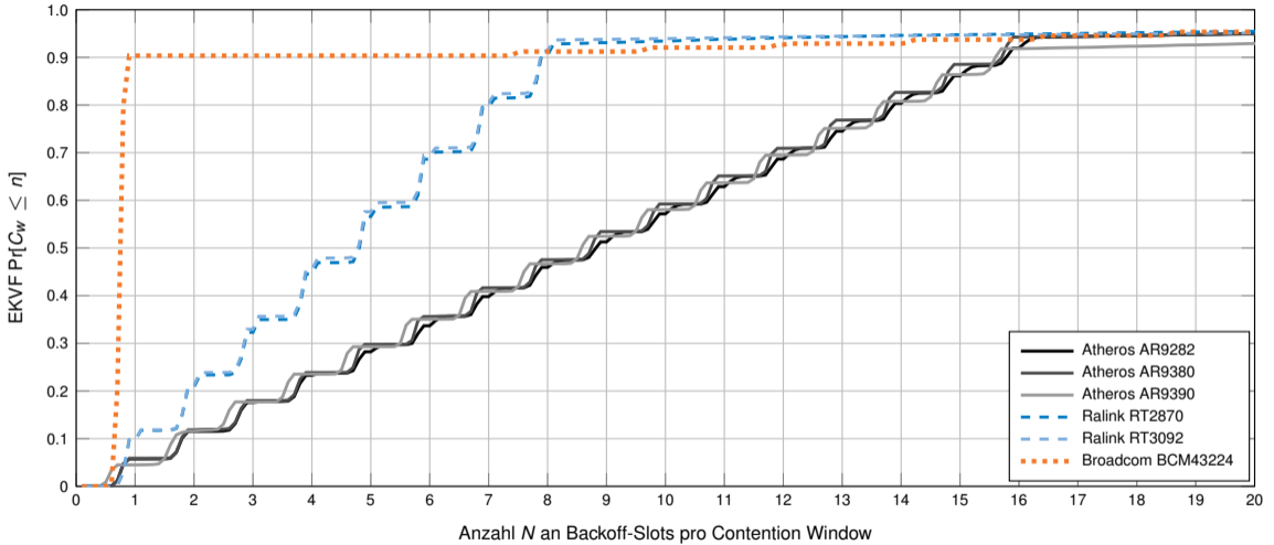
EKFV der zeitl. Abstände zwischen Frames einer Station gemessen in Vielfachen von Slotzeiten.
