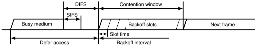
Abbildung 3: IEEE 802.11 DCF
