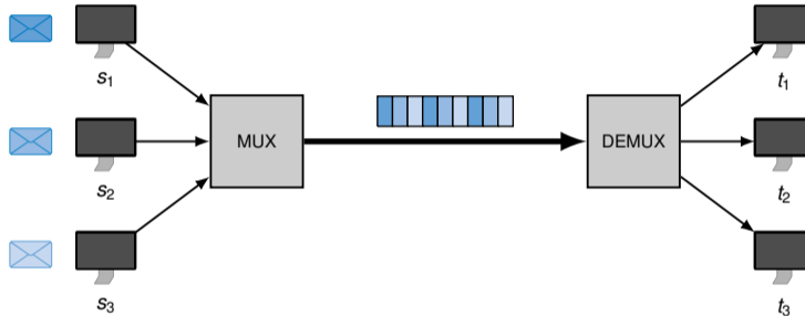
Abbildung 2: Deterministisches Zeitmultiplex-Verfahren
