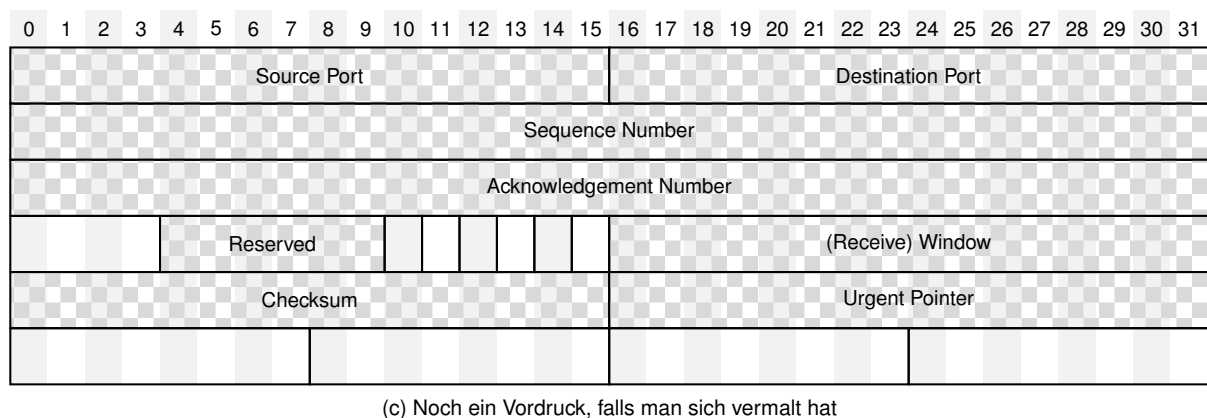
Abbildung 3.1: TCP-Header und Vordrucke zur Lösung von Aufgabe 3
